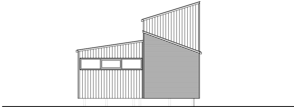
ELEVATION B
