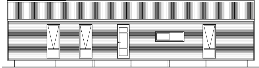
ELEVATION A
